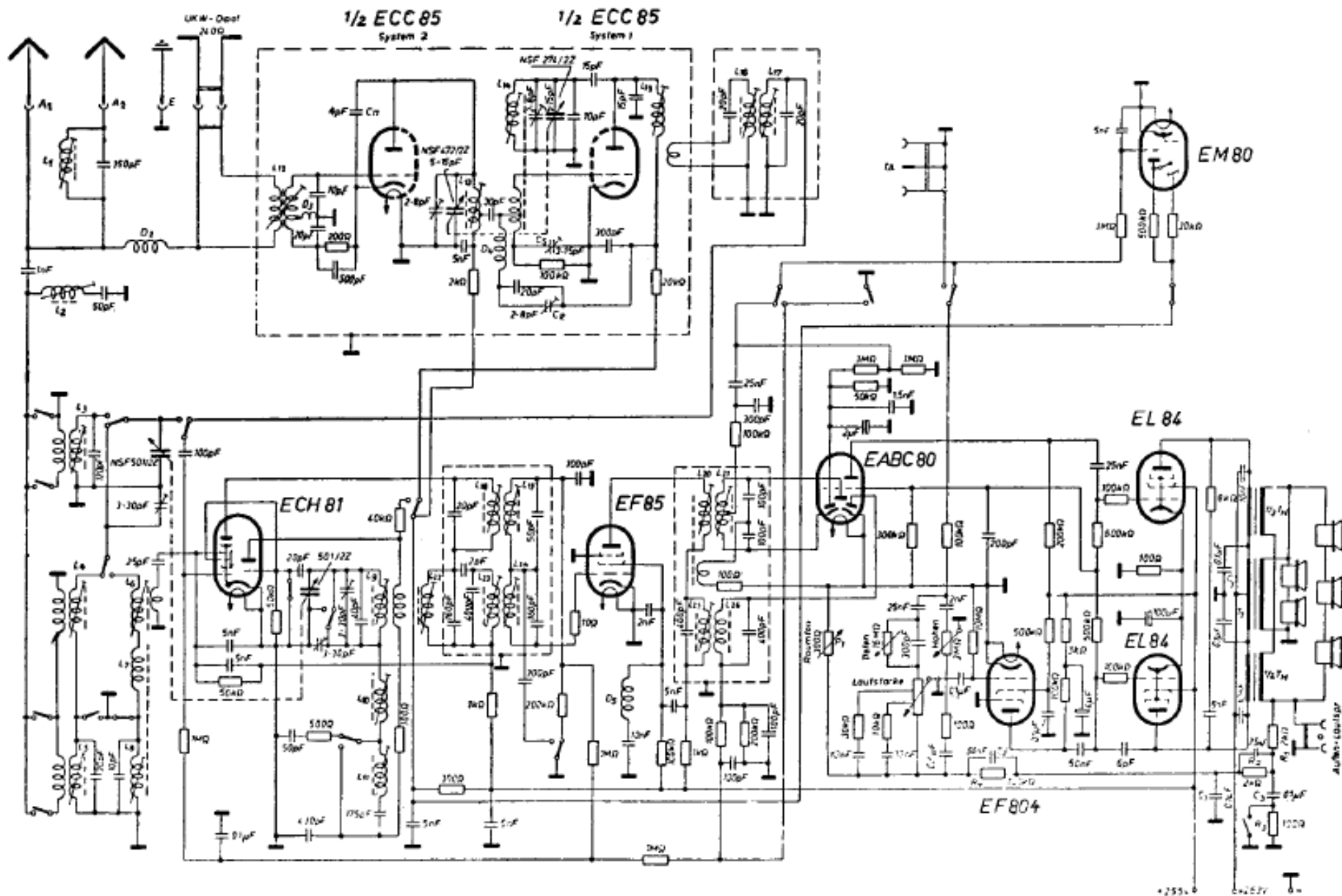
CONTINENTAL (Continental-Rundfunk GmbH, Osterode, Harz) - Mod. Imperial 450 Stereo) - Ricevitore a modulazione di ampiezza e di frequenza. Onde lunghe da 140 a 375 kc/s, onde medie da 510 a 1700 kc/s, onde corte da 5,8 a 12,6 Mc/s, onde ultracorte FM da 87,5 a 100,5 Mc/s. Tipo a soprammobile con riproduzione stereofonica mediante cinque altoparlanti, due grandi, due medi laterali ed uno piccolo centrale. (Alimentatore non disegnato). Prod. 1956.
